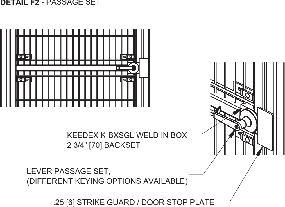
DETAIL F2 - PASSAGE SET
